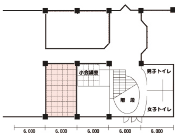
ホール図面
